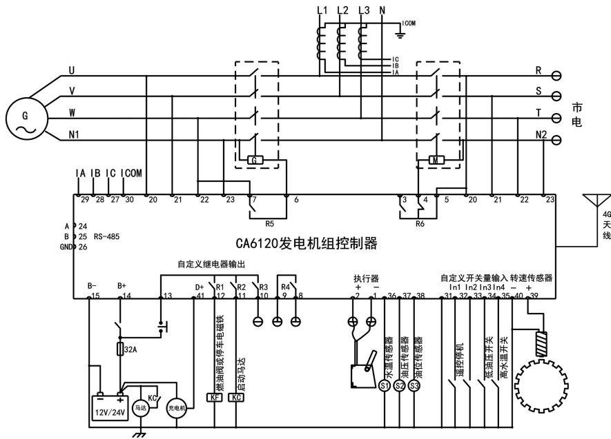
图 5 单机自启动 ATS 接线图
