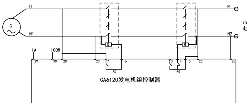
图 6 单相两线制接线图
