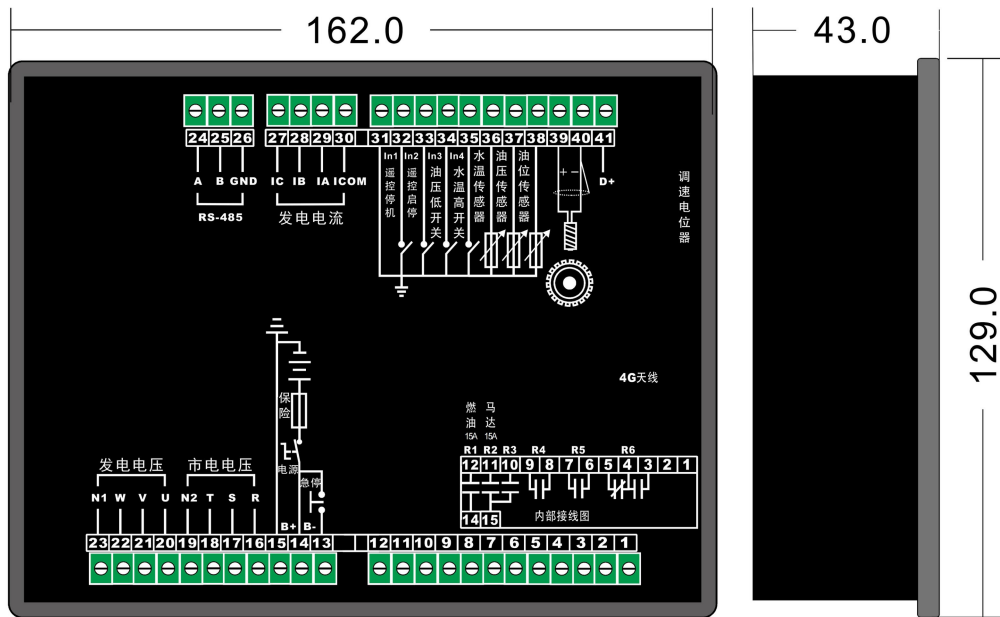
图 9 外形及开孔尺寸图
