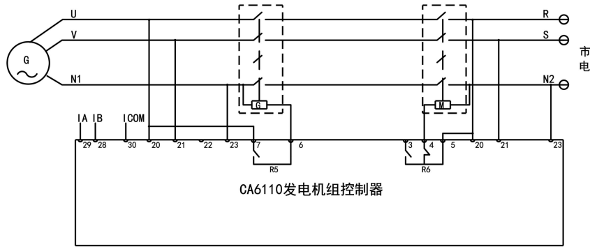
图 7 单相三线制接线图
