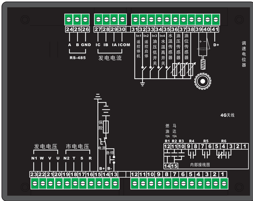
图 2 控制器接线端子图
