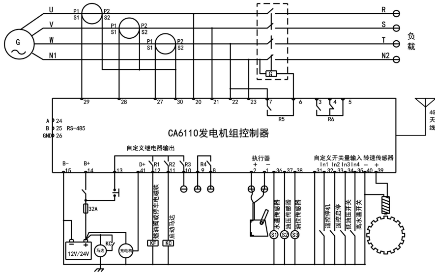
图 4 单机自启动接线图
